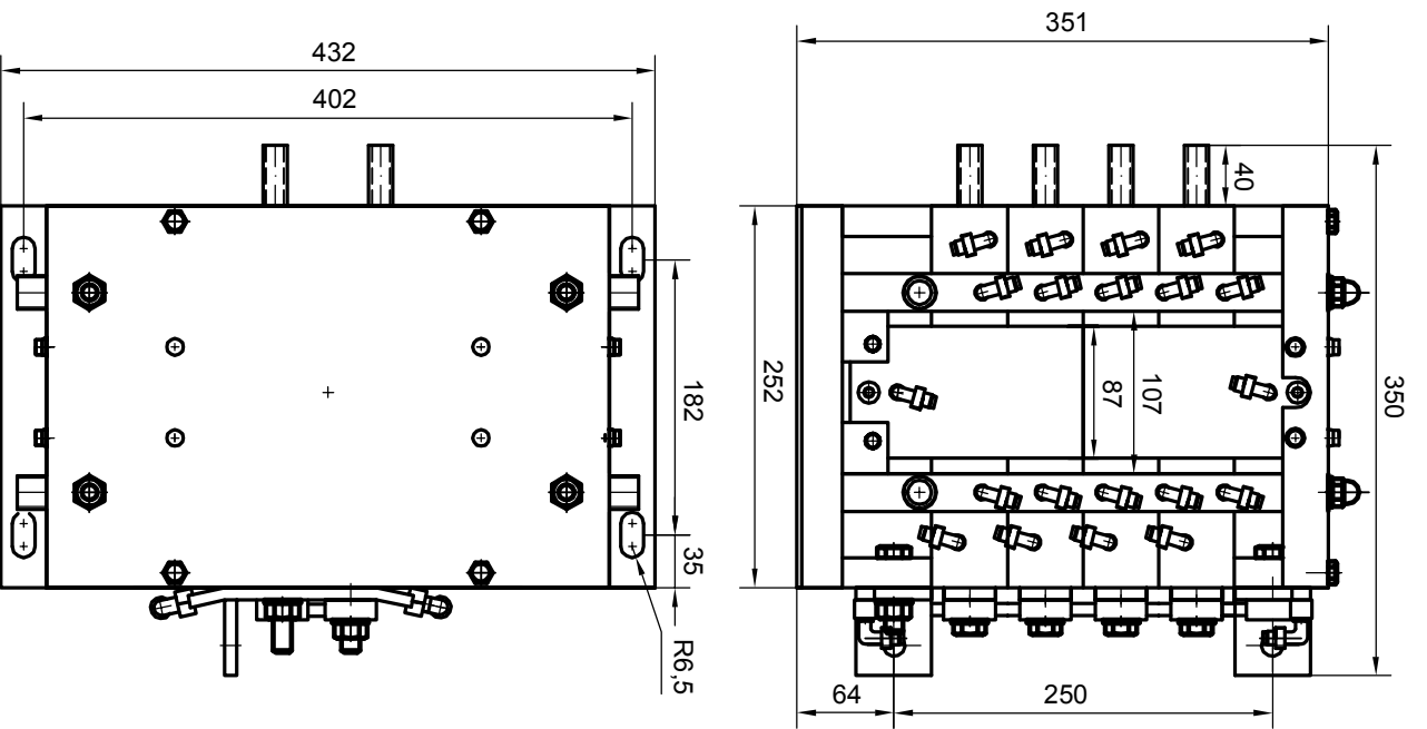
Габаритные и установочные размеры трансформатора ТЗ1-1600С4 масса трансформатора - 85 кг.
