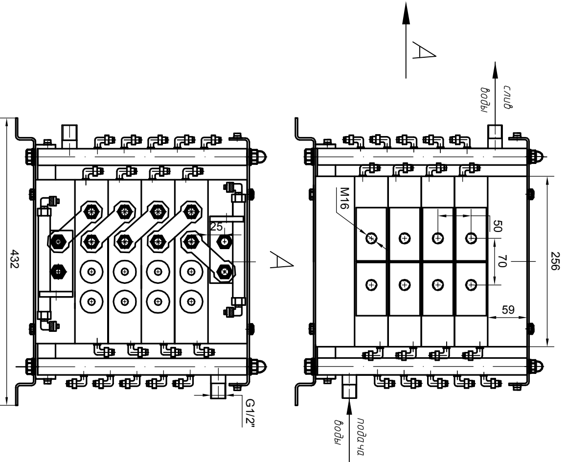
Габаритные и установочные размеры трансформатора ТЗ1-1600С4 масса трансформатора - 85 кг.
